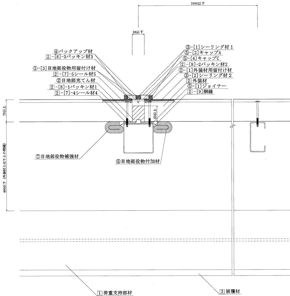
水平断面詳細図 (FP060NE-0162-2) (タイプ7)
