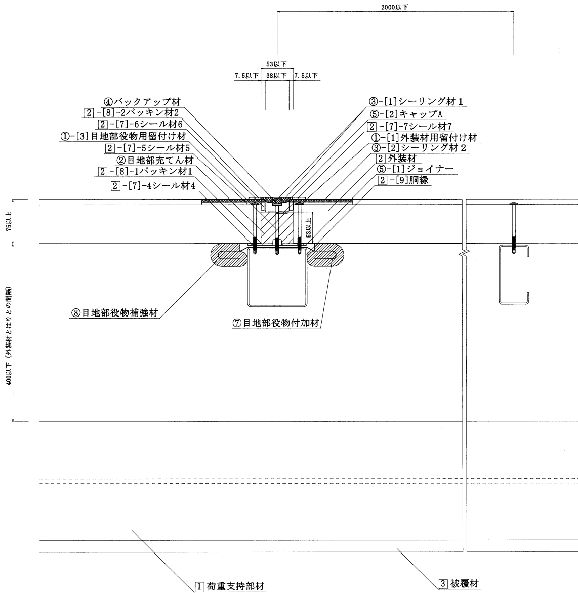
水平断面詳細図 (FP060NE-0162-2) (タイプ 2)
