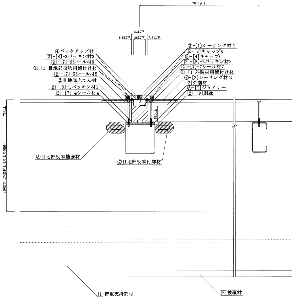
水平断面詳細図 (FP060NE-0162-2) (タイプ 4)
