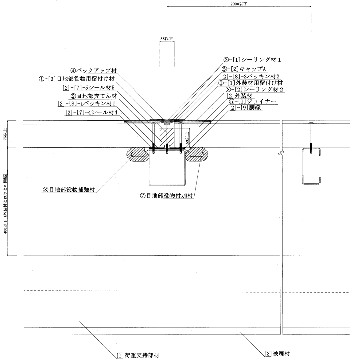
水平断面詳細図 (FP060NE-0162-2) (タイプ5)
